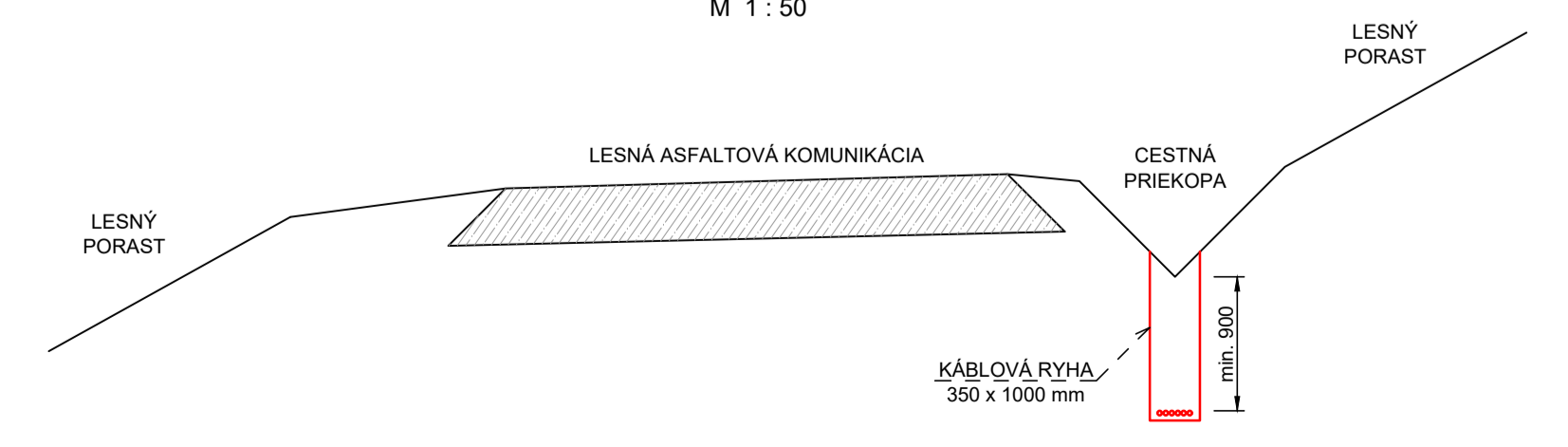
VZOROVÝ REZ LESNOU ASFALTOVOU KOMUNIKÁCIOU S UMIESTNENÍM TRASY NAVRHOVANÝCH OPTICKÝCH VEDENÍ M 1 : 50
