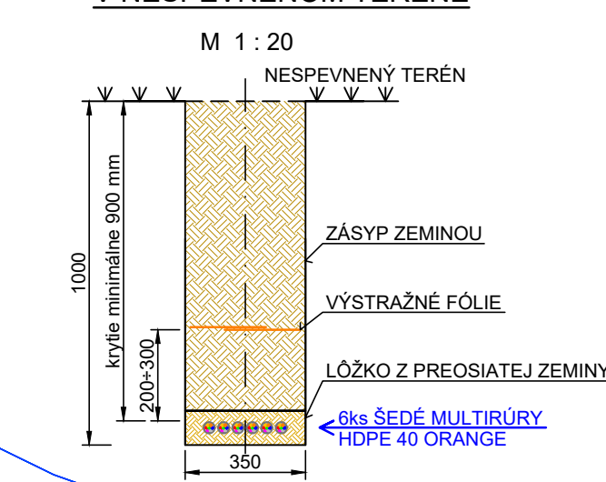
REZ KÁBLOVOU RYHOU V EXTRAVILÁNE V NESPEVNENOM TERÉNE
