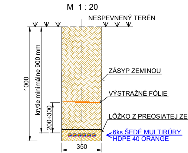
REZ KÁBLOVOU RYHOU V EXTRAVILÁNE V NESPEVNENOM TERÉNE
