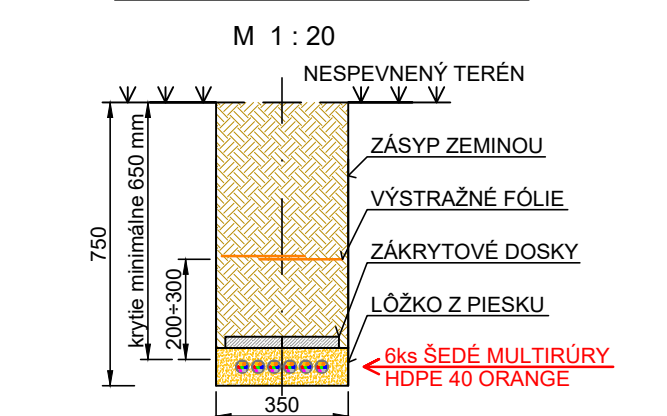
REZ KÁBLOVOU RYHOU V INTRAVILÁNE V NESPEVNENOM TERÉNE
