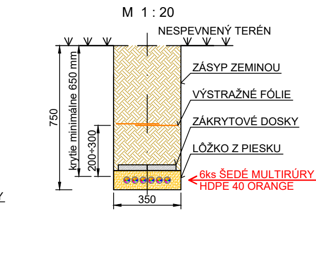
REZ KÁBLOVOU RYHOU V INTRAVILÁNE V NESPEVNENOM TERÉNE
