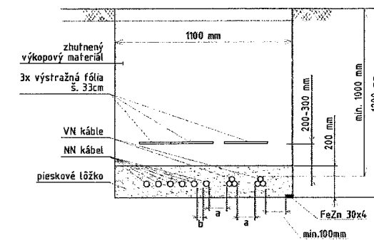
SPOLOČNÁ TRASA VN A NN - VOLNÝ TERÉN
