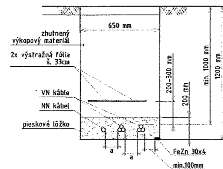
SPOLOČNÁ TRASA VN A NN - VOLNÝ TERÉN
